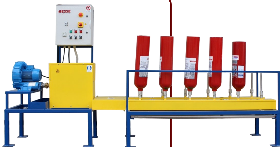
Versione 6 posti con collettore dal basso
